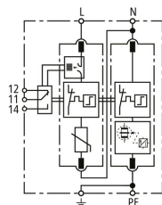
Schéma de principe du circuit DG M TT 2P ACI 275 FM
