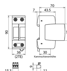
Dimensions DG M TT 2P ACI 385 FM
