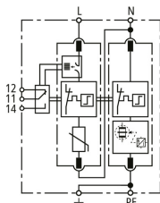
Schéma de principe du circuit DG M TT 2P ACI 385 FM
