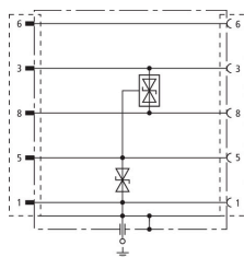
Schéma de principe du circuit FS 9E PB 6
