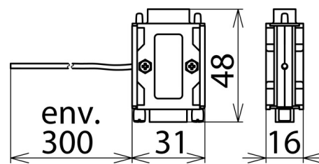
Dimensions FS 9E PB 6
