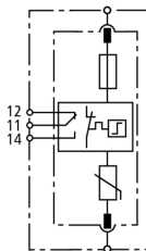
Esquema del DG SE CI 440 FM
