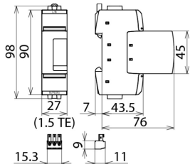
Dimensiones del DG SE CI 440 FM
