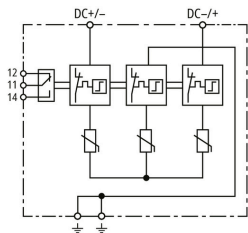
Schema di principio DCU 2 YPV 1+2 1000 1M 2S FM
